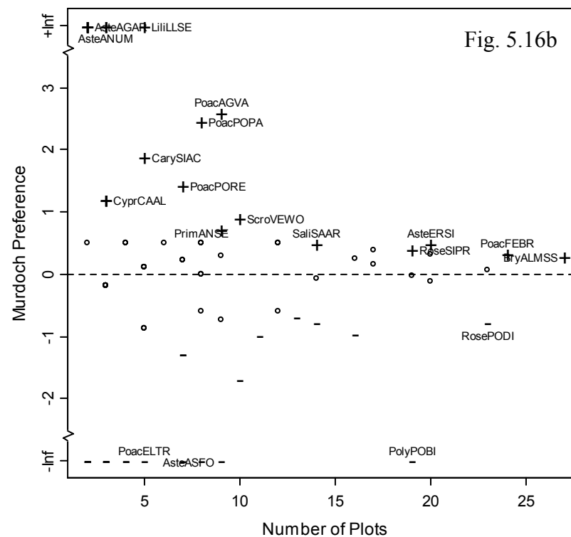
N. Absaroka Snowbank
