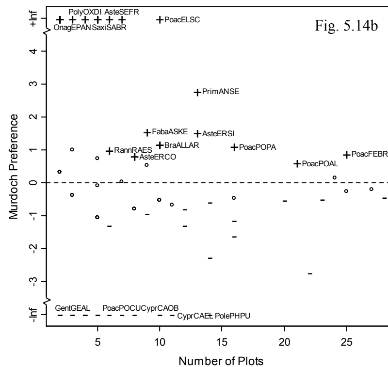
N. Absaroka N. face
