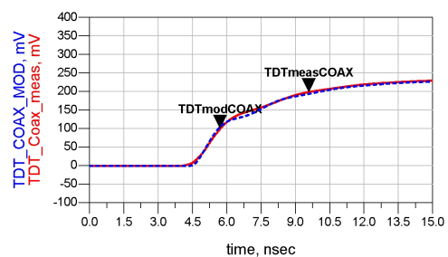
(d) Coax Cable TDT
